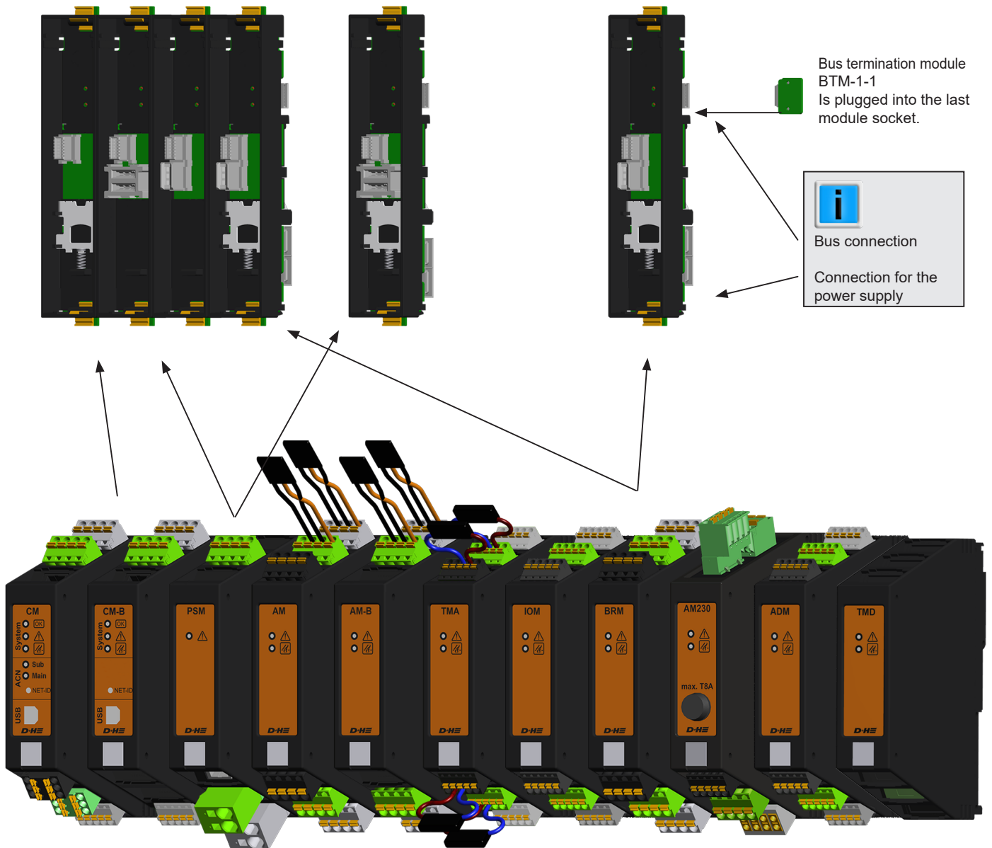
Basic module socket MS-D1-RR-TS
